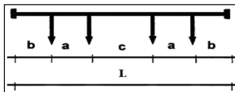
Figura 5.48 – Modelli di carico realmente circolanti (UIC-code 700). Schema geometrico di un carro.
