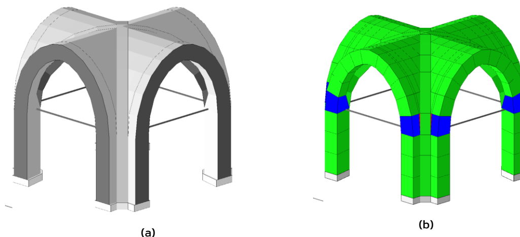
Figura 4.2 - A sinistra (a) vista del modello geometrico di una volta a crociera; a destra (b) vista del modello computazionale equivalente.
