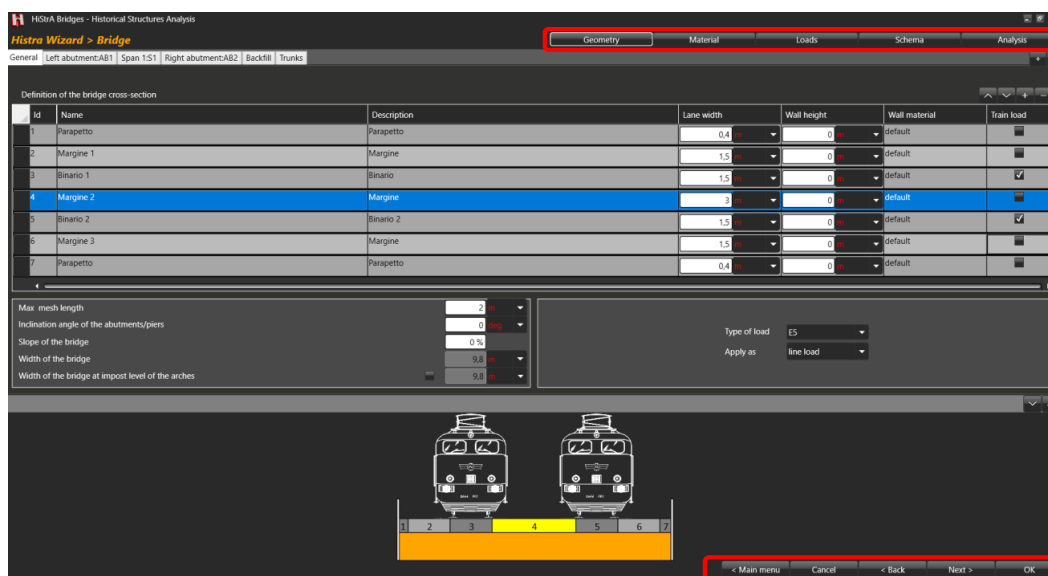
Figura 5.2 - Schermata generale Wizard di HISTRA BRIDGES, per l'input geometrico di un ponte ferroviario – Rail Bridge
