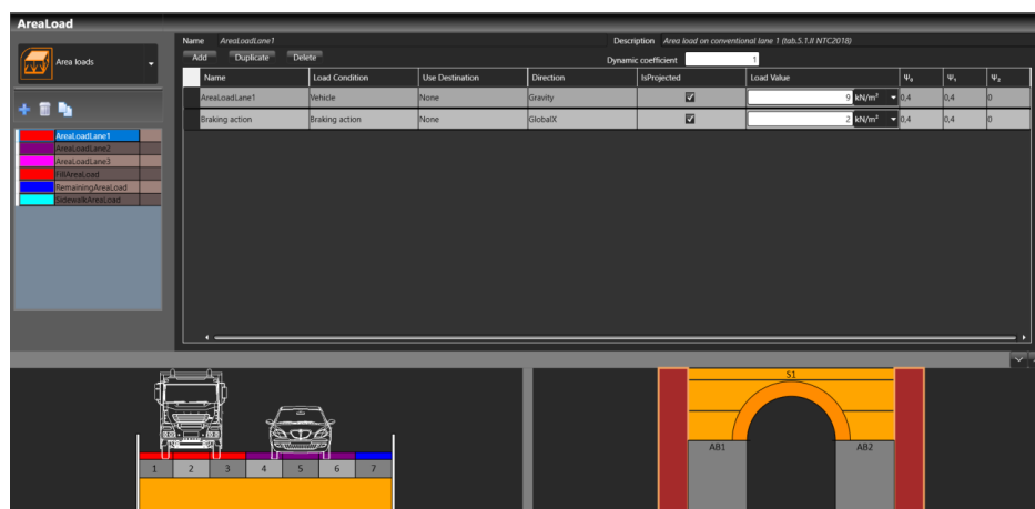
Figura 5.58 - Definizione dei Carichi di Area - Area Loads - Esempio carico veicolare e azione frenante su ponti stradali.
