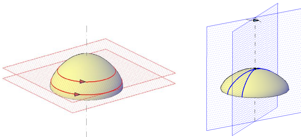
Figura 2.9 - Generatrici e direttrici di una cupola.
