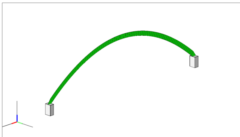
Figura 7.23 – Esempio Modello computazionale e piano medio elementi Quad.
