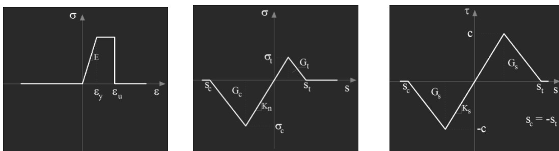
Figura 5.43 - Legame costitutivo materiale FRP
