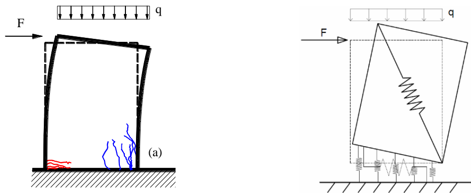
Figura 5.31 – a) Meccanismo di rottura a flessione di un pannello murario; a') Attivazione del meccanismo di rocking sul macro-elemento a quattro nodi di HISTRA
