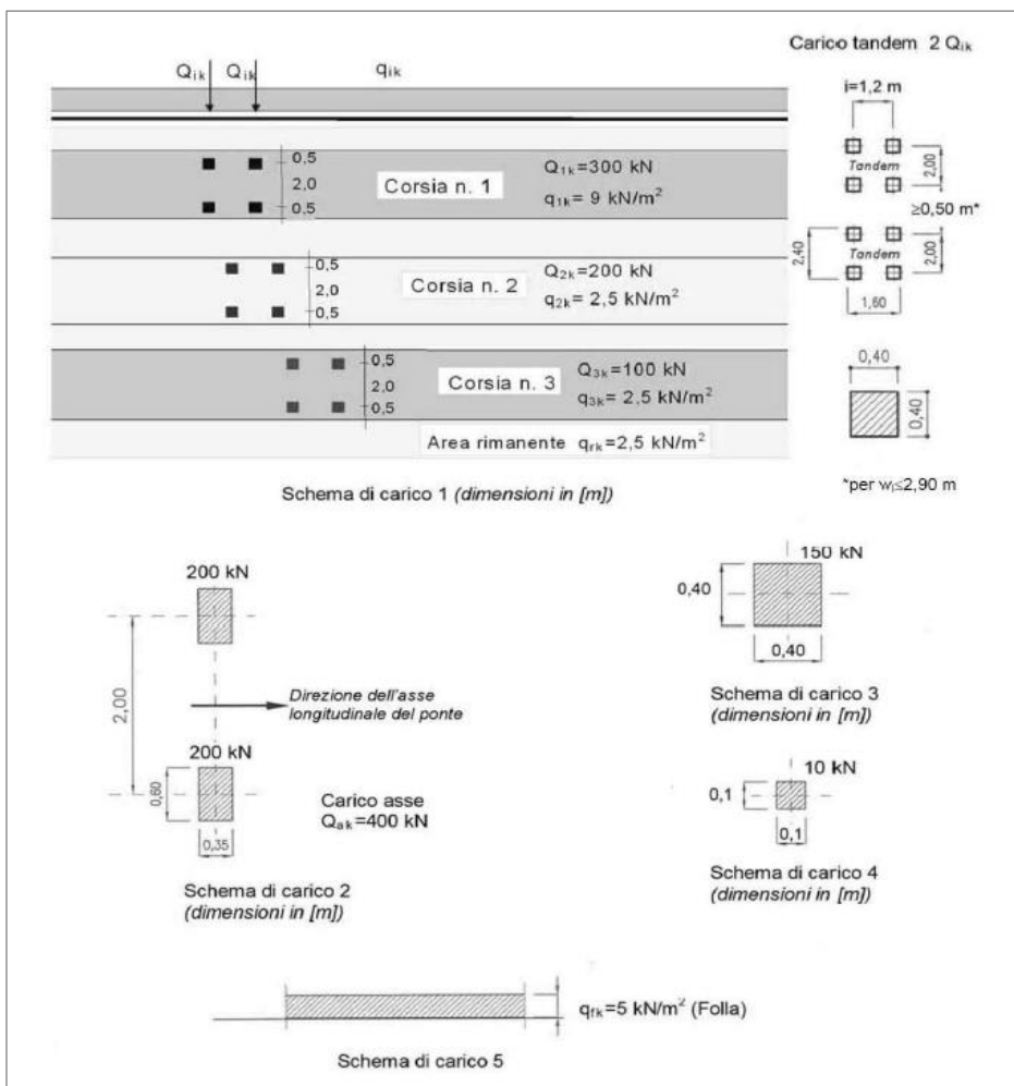
Figura 5.14 – Disposizione dei carichi mobili - Schemi di carico 1 – 5 (dimensioni in m) – Figura 5.1.2 delle NTC2018
