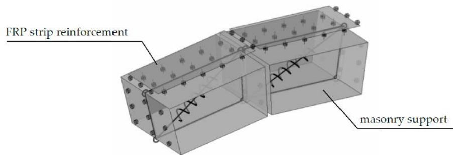
Figura 2.4 – Strategia di modellazione del rinforzo di volte in muratura mediante applicazione di FRP
