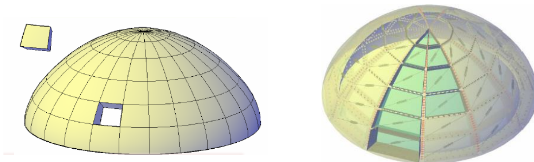
Figura 2.1 - A sinistra (a) suddivisione di una cupola in porzioni omogenee; a destra (b) modello a macro-elementi equivalente
