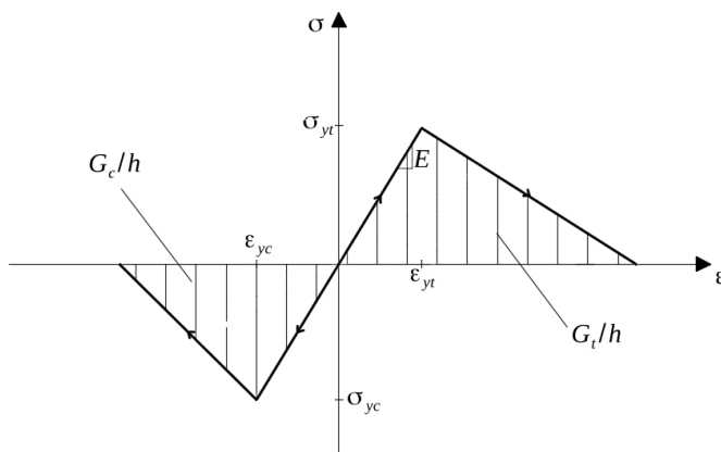
Figura 5.34 – Individuazione della energia di frattura nel caso di legame costitutivo elastico con softening lineare
