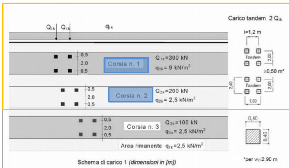
Figura 5.54 – Esempio carichi veicolari schema di carico 1 NTC2018 – figura 5.12 – Schema di carico1.
