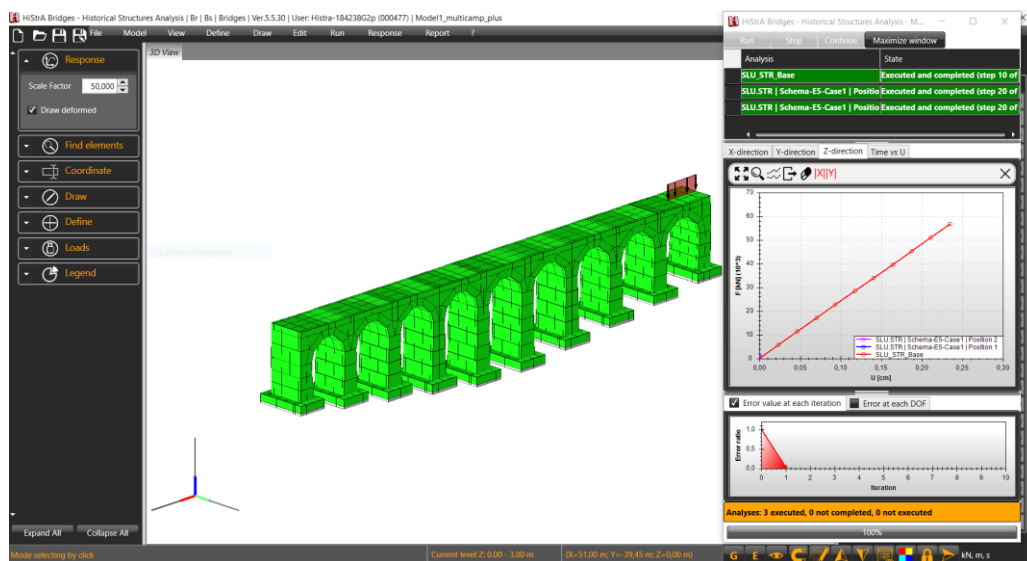
Figura 7.57 – Finestra di esecuzione delle analisi e visualizzazione del modello tridimensionale.
