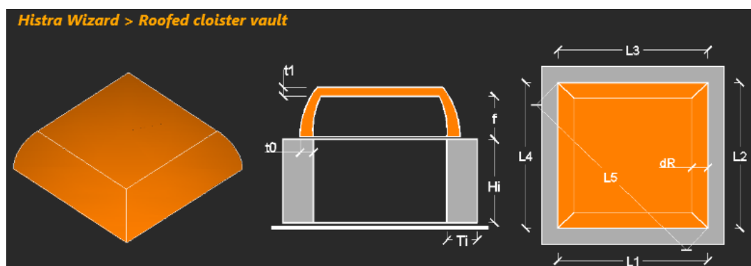
Figura 4.14 - Schermata di riferimento per la creazione del modello geometrico di una volta a specchio
