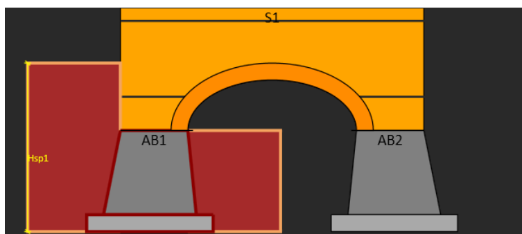
Figura 5.17 - Rappresentazione grafica della sezione trasversale del ponte e caratterizzazione della altezza spinta terreno a monte e a valle
