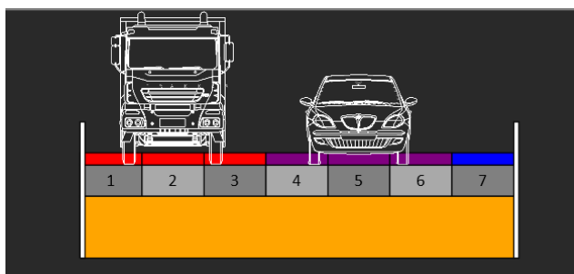
Figura 5.11 – Esempio di definizione della sezione trasversale, per ponti stradali
