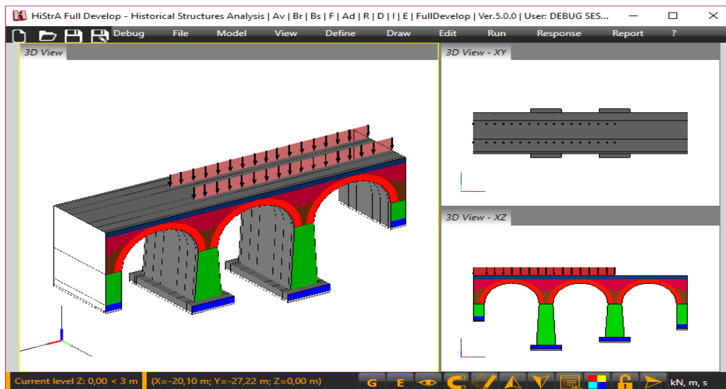
Figura 5.49 – Modellazione mediante carichi lineari equivalenti (Line Load).
