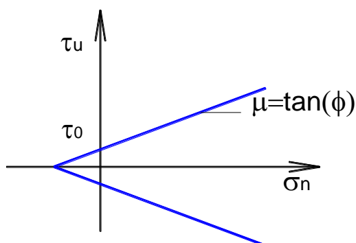
Figura 5.39 – Legame costitutivo per meccanismo di rottura a taglio per scorrimento all'interfaccia
