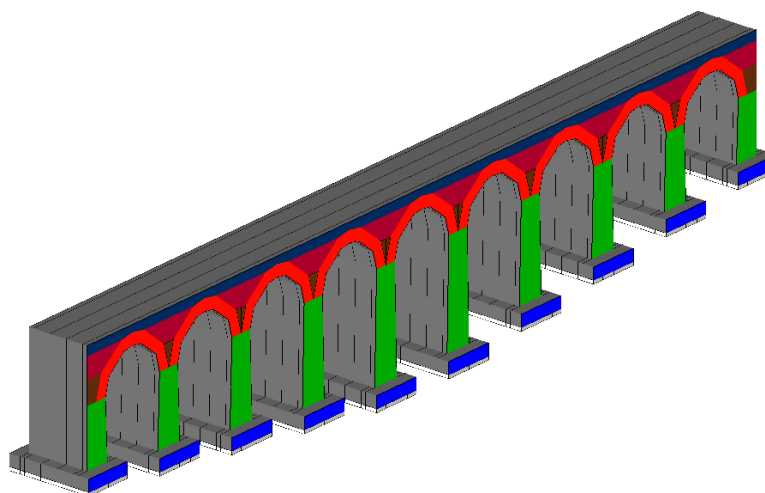
Figura 7.13 – Vista del modello geometrico
