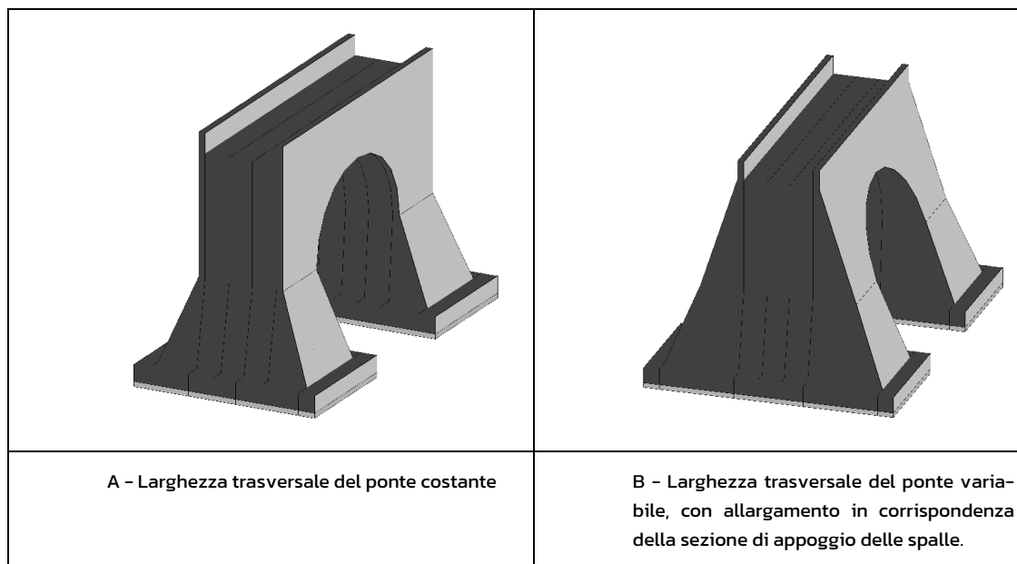
Figura 5.9 – Caratterizzazione della larghezza trasversale del ponte
