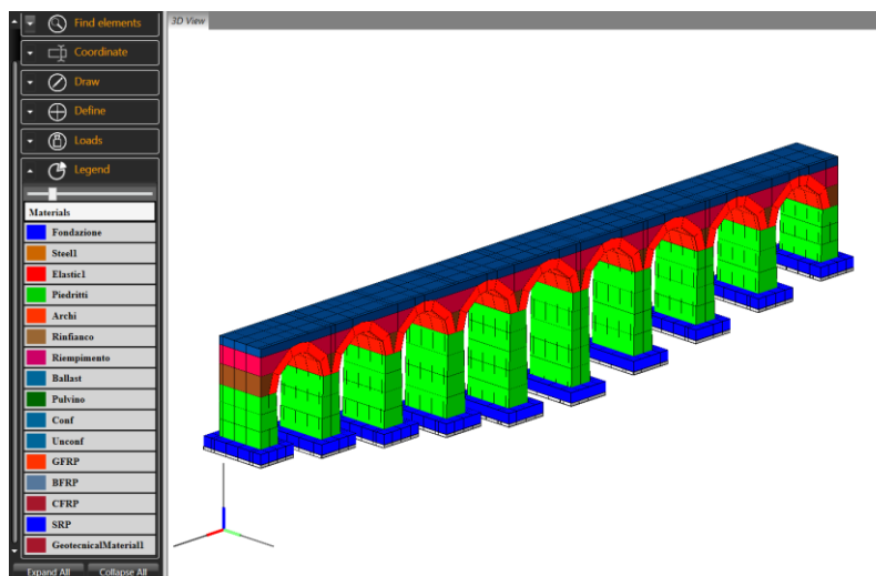
Figura 7.19 – Visualizzazione del modello e degli elementi, colorati in funzione dei materiali assegnati
