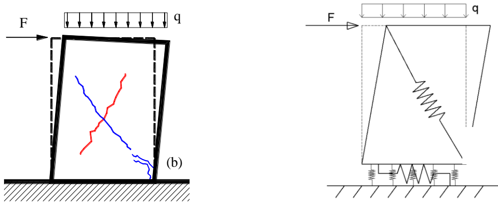
Figura 5.35 – b) Meccanismo di rottura per fessurazione diagonale; b') Attivazione del meccanismo sul macro-elemento a quattro nodi di HISTRA
