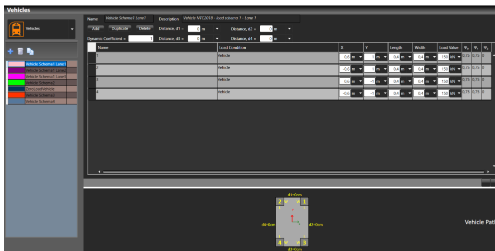
Figura 7.21 – Esempio definizione carichi veicolari per ponte stradale.
