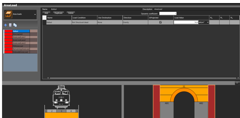
Figura 5.57 - Definizione dei Carichi di Area - Area Loads - Esempio carico di area per ponti ferroviari.
