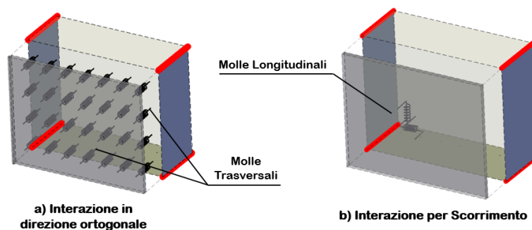
Figura 2.5 – Interazione in direzione normale e per scorrimento all’interfaccia tra rinforzo e support in muratura.
