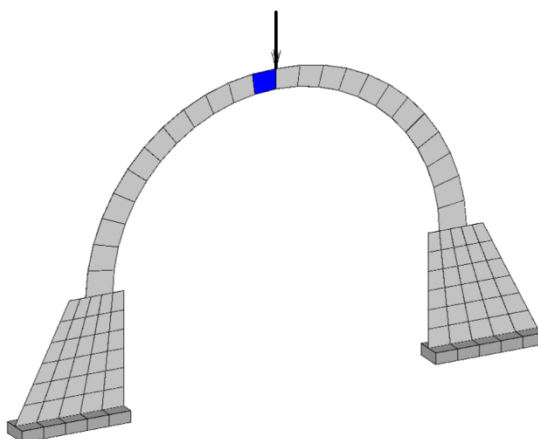
Figura 7.32 – Visualizzazione di un arco caricato da una forza concentrata in sommità sulla sezione di chiave
