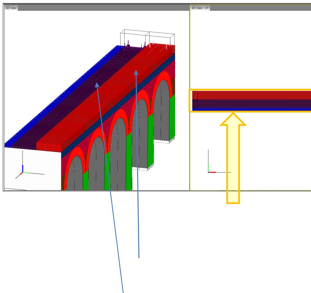
Figura 5.53 – Visualizzazione del modello 3d del ponte e dei carichi veicolari - schema 1
