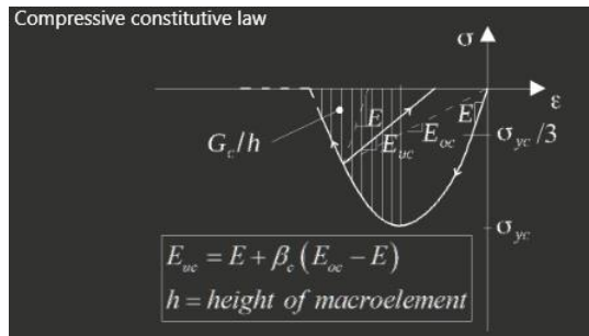
E) Parabolic: legame costitutivo di tipo non lineare con legge parabolica, calibrato in funzione dell'energia di frattura
