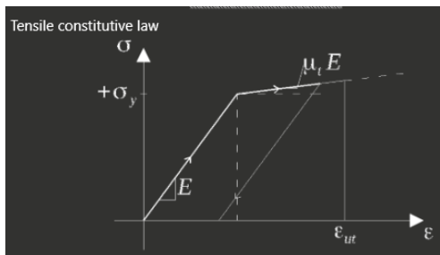
B1) Linear hardening - legame costitutivo a trazione di tipo elasto-plastico con incrudimento cinematico lineare e duttilità fissata
