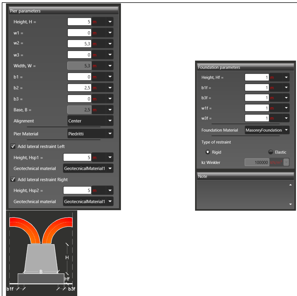
Figura 5.22 - Pile N - input delle proprietà geometriche della pila.
