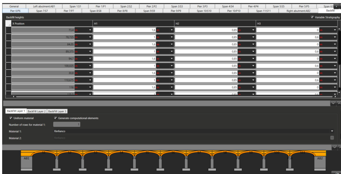
Figura 5.24 - Scheda Backfill - input delle proprietà del profilo stratigrafico di rinfianchi e riempimento.
