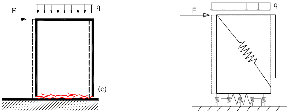
Figura 5.38 - c) Meccanismo di rottura a taglio per scorrimento; c') Attivazione del meccanismo sul macro-elemento a quattro nodi di HISTRA
