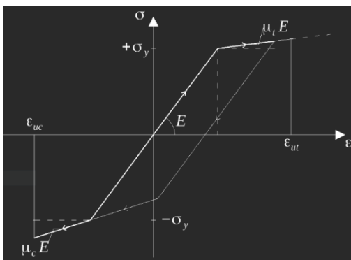
Figura 5.41 - Legame costitutivo acciaio
