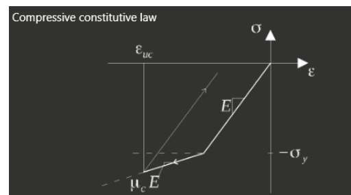
B2) Linear hardening - legame costitutivo a compressione di tipo elasto-plastico con incrudimento cinematico lineare e duttilità fissata
