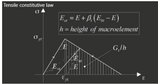
C) Linear softening - Legame costitutivo elastico con softening lineare calibrato in funzione dell'energia di frattura
