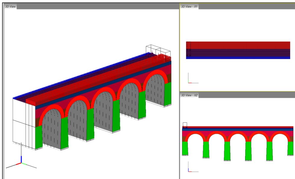
Figura 5.53 – Visualizzazione del modello 3d del ponte e dei carichi veicolari - schema 1
