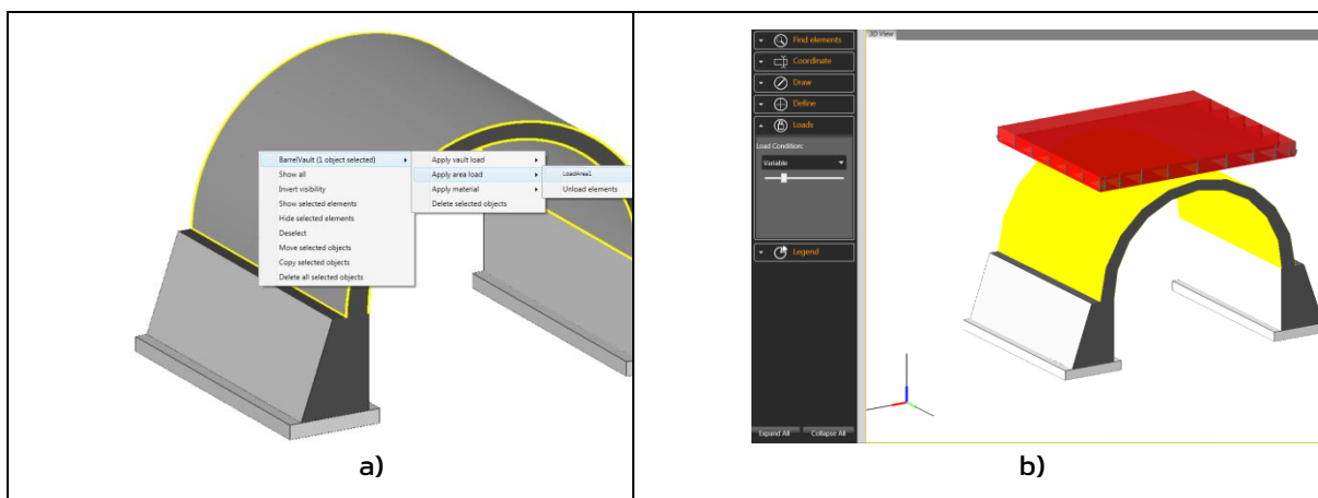
Figura 7.26 – a) Assegnazione di un carico di area ad una volta a botte; b) Visualizzazione del carico di area assegnato (visualizzazione dei carichi appartenenti alla condizione di carico selezionata)
