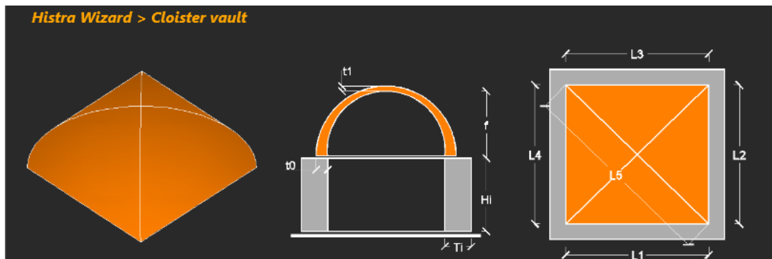
Figura 4.12 – Schermata di riferimento per la creazione del modello geometrico di una volta a padiglione
