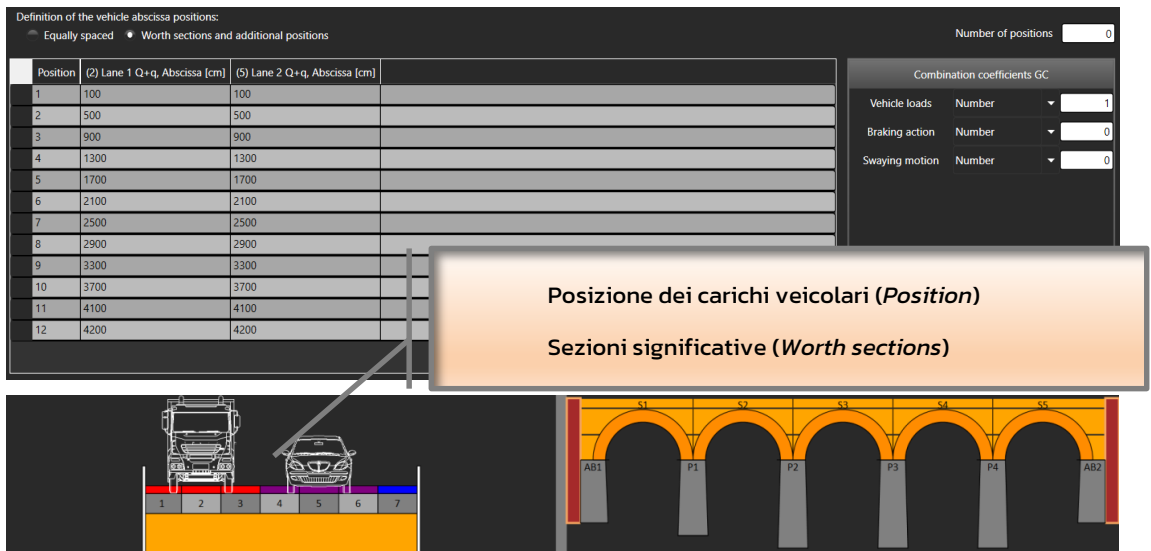
Figura 5.65 – Posizioni dei carichi viaggianti. Esempio ponte stradale.
