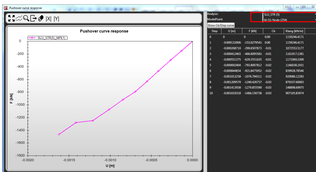
Figura 7.64 – Curva di push-over F-U
