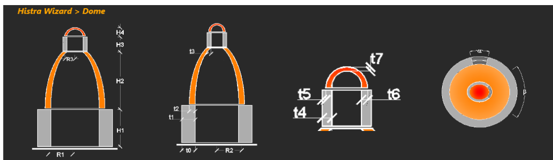
Figura 4.16 – Schermata di riferimento per la creazione del modello geometrico di una cupola
