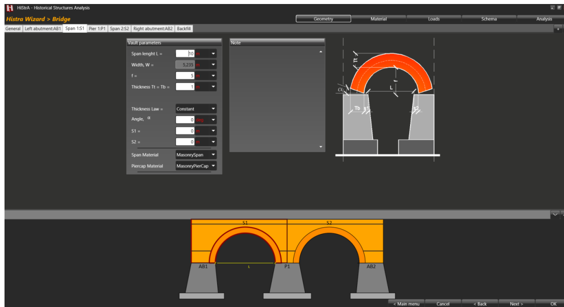
Figura 5.20 – Scheda Span 'N' – input delle proprietà geometriche della campata n-esima del ponte ( Vault parameters ).
