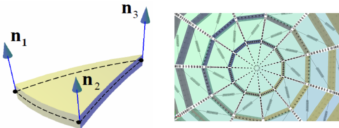
Figura 2.3 – Macro-elemento a 3 nodi
