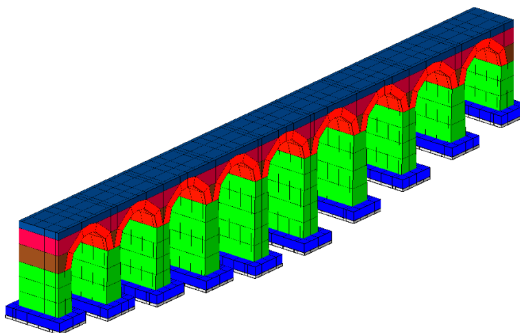
Figura 7.14 – Vista del modello computazionale
