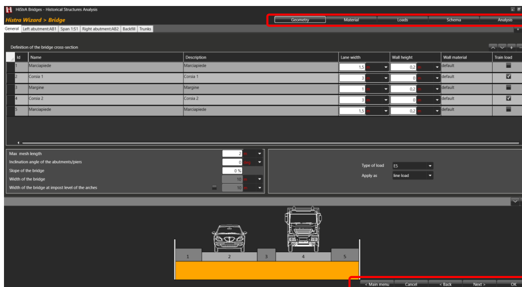
Figura 5.3 - Schermata generale Wizard di HISTRA BRIDGES, per l'input geometrico di un ponte stradale – Road Bridge
