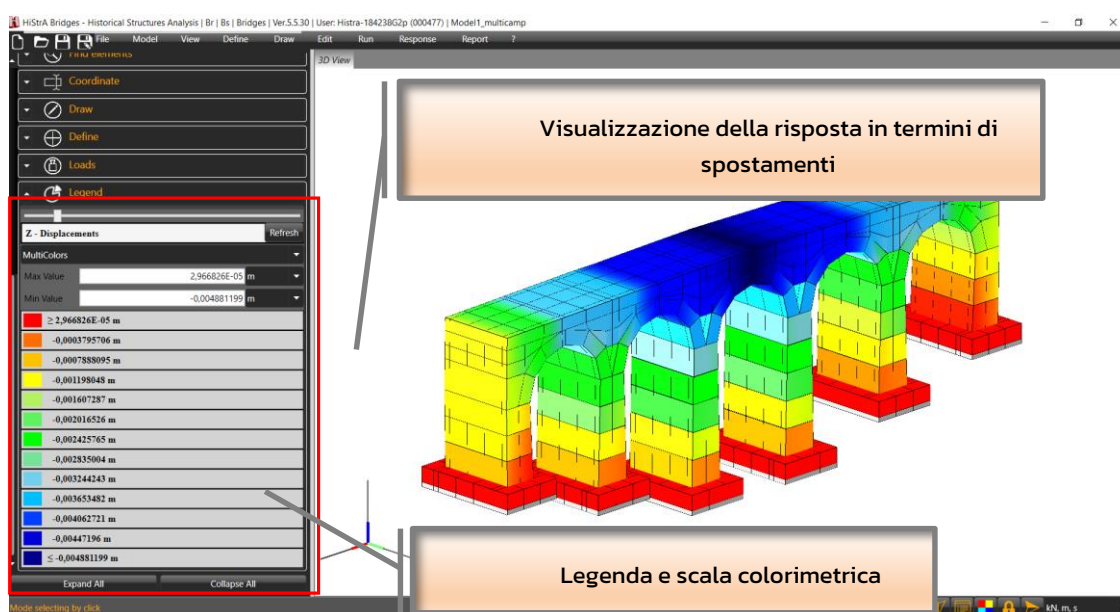
Figura 7.60 – Response – Visualizzazione della risposta in termini di spostamenti
