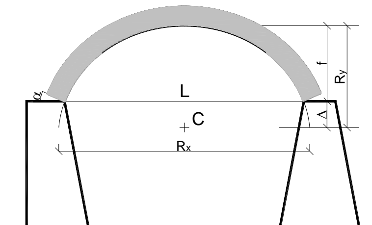
Figura 5.21 - Schema geometrico della sezione della volta.
