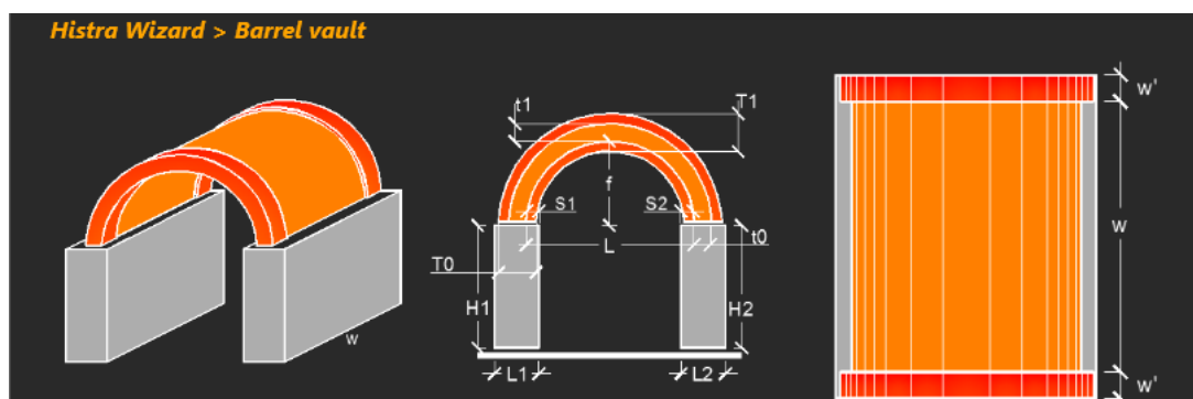
Figura 4.6 – Schermata di riferimento per la creazione del modello geometrico di una volta a botte
