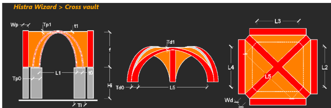
Figura 4.8 - Schermata di riferimento per la creazione del modello geometrico di una volta a crociera
