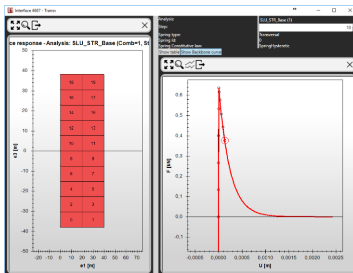
Figura 7.62 - Finestra di visualizzazione della risposta delle molle di interfaccia: curva di carico
