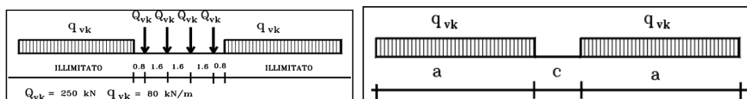
Figura 5.47 – Modelli di carico teorici, adottati in fase di progettazione di nuove strutture (LM71, per il traffico normale e SWO e SW2 per il traffico pesante).
