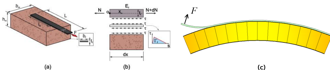
Figura 2.7 – a) e b) Scorrimento del rinforzo sulla muratura, c) Distacco per sollevamento del rinforzo dalla muratura di support
