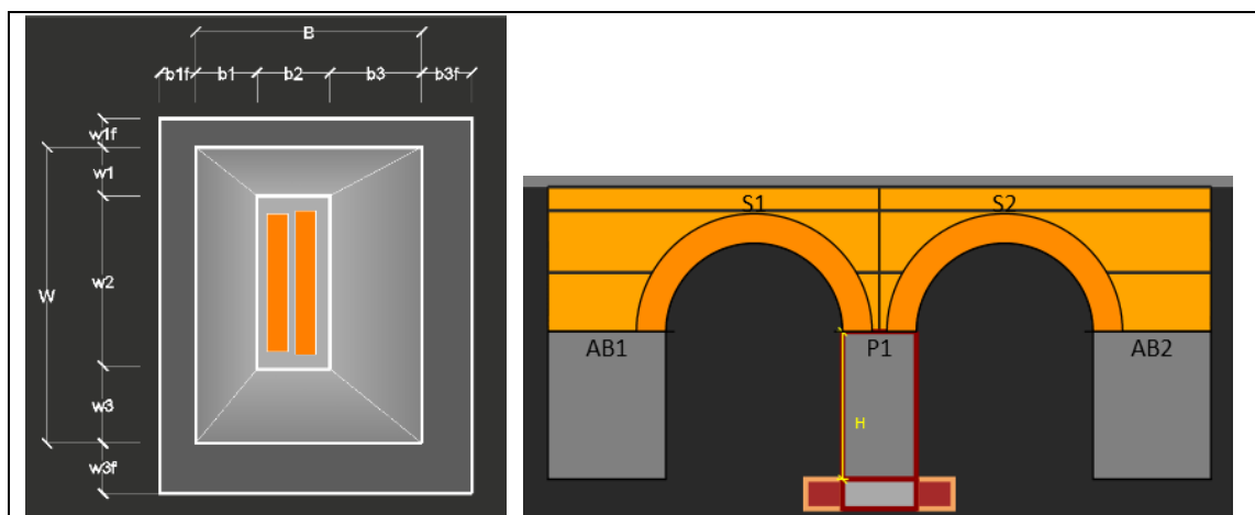
Figura 5.23 - Pile N - input delle proprietà geometriche della fondazione della pila e vista trasversale del ponte.
