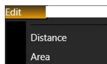
Figura 7.53– Menu EDIT
