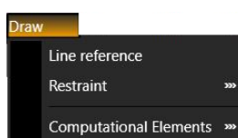
Figura 7.51 – Menu DRAW.
