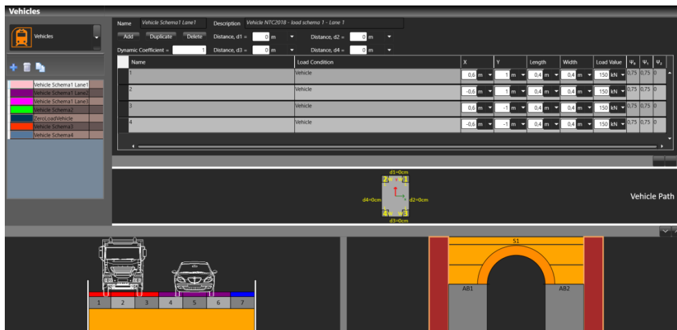
Figura 5.51 – Definizione dei carichi veicolari, modellati come carichi concentrati su due assi in tandem (Vehicle load).
