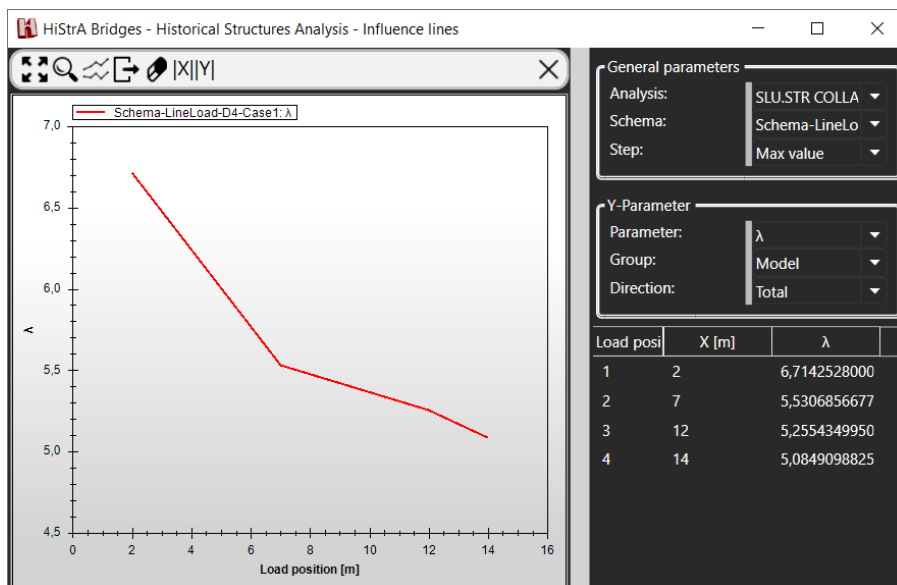
Figura 7.67 – Finestra “Influence Lines” per la visualizzazione delle linee di influenza
