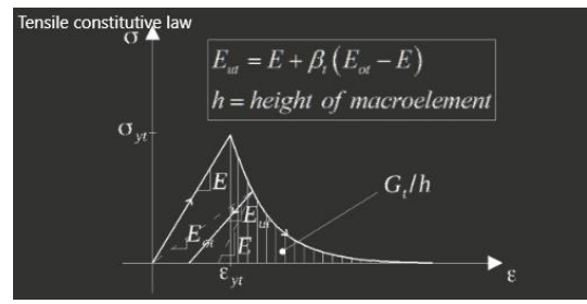
D) Exponential softening - legame costitutivo elastico con softening non lineare calibrato in funzione dell'energia di frattura
