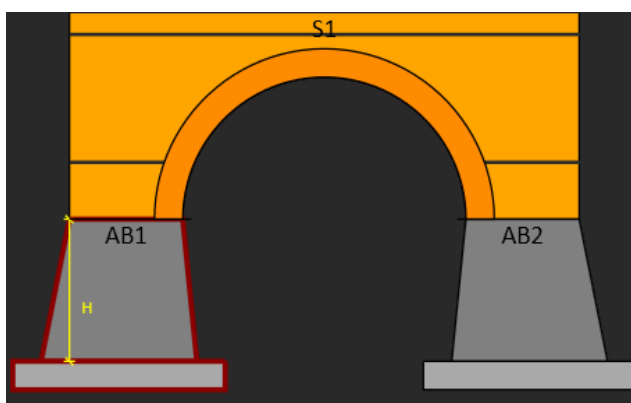
Figura 5.16 – Rappresentazione grafica della sezione trasversale del ponte e individuazione interattiva dei parametri geometrici della spalla
