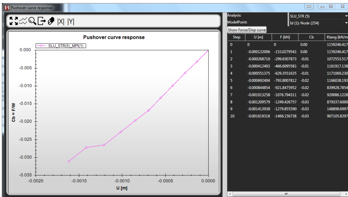
Figura 7.65 – Curva di push-over in termini di moltiplicatore dei carichi -spostamento \lambda-U
