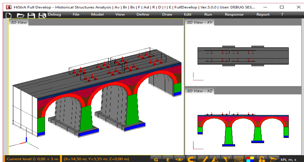
Figura 5.50 – Modellazione mediante carichi concentrati (Vehicle Load)
